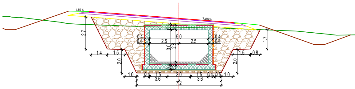
ПОПРЕЧНИ ПРЕСЕК САНДУЧАСТОГ ПРОПУСТА
