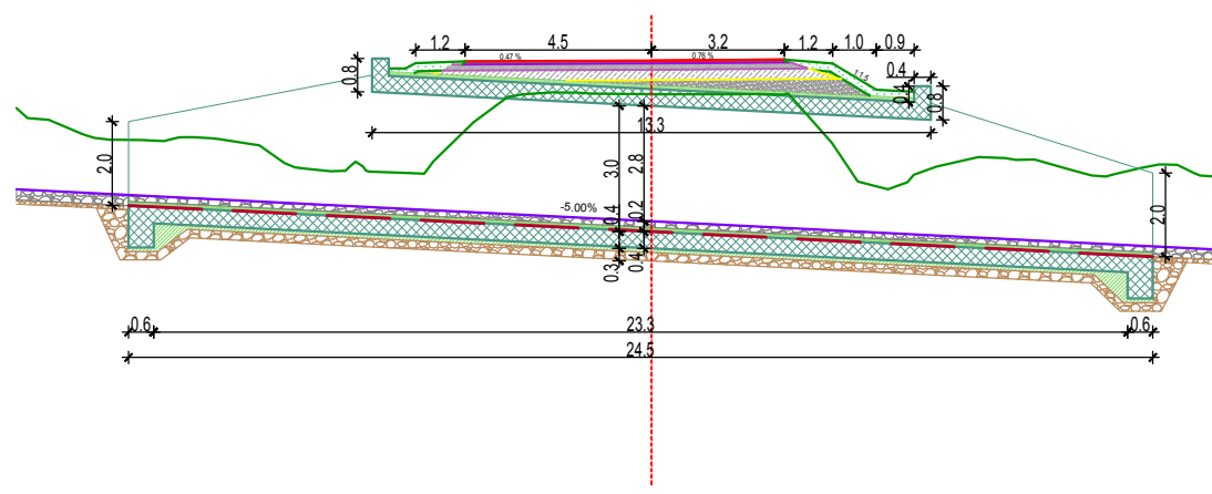
ПОДУЖНИ ПРЕСЕК САНДУЧАСТОГ ПРОПУСТА
